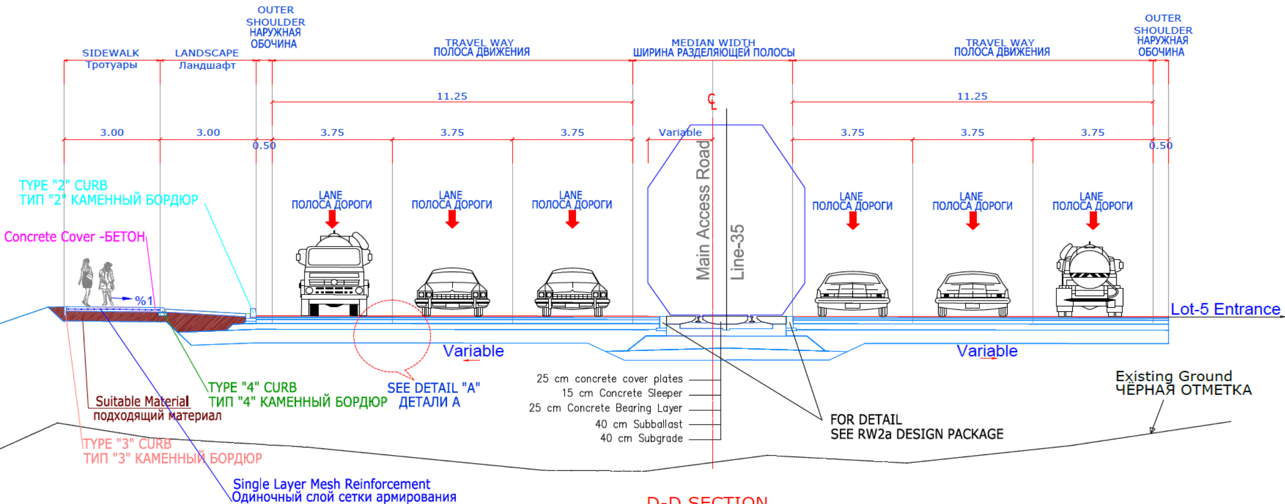
D-D SECTION РАЗРЕЗ D-D
