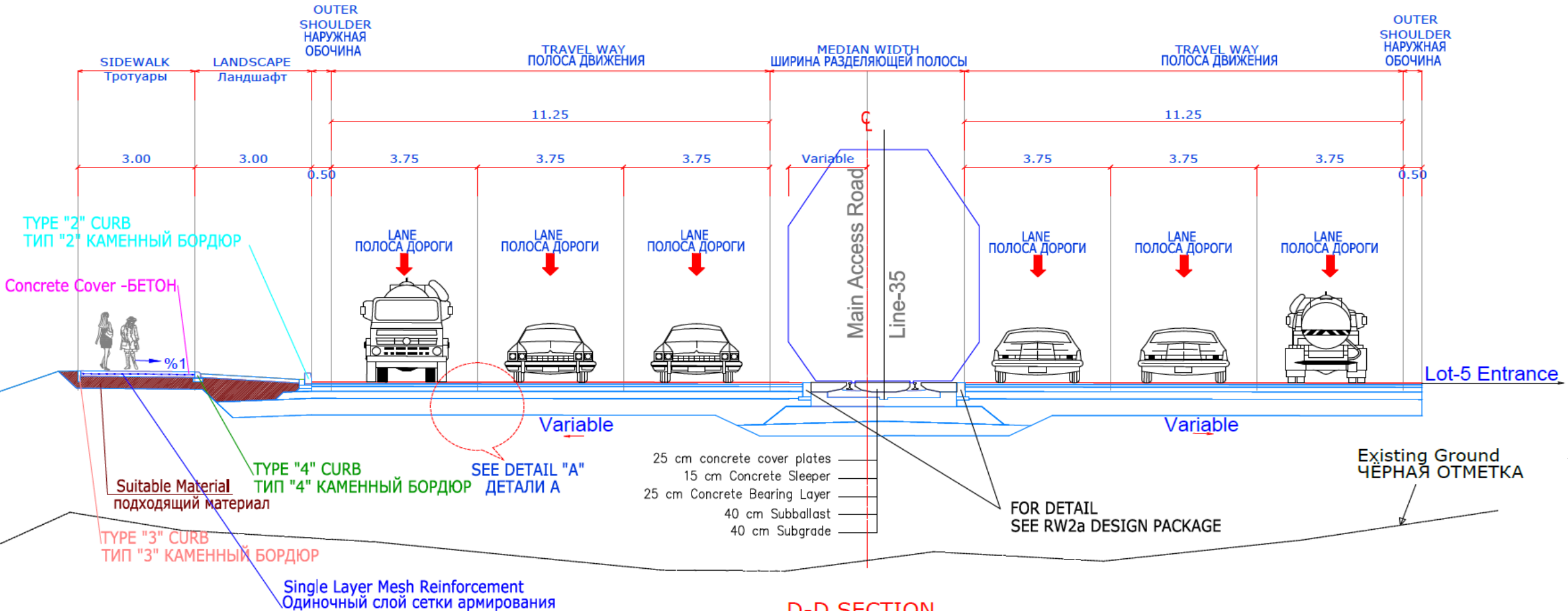
D-D SECTION РАЗРЕЗ D-D
